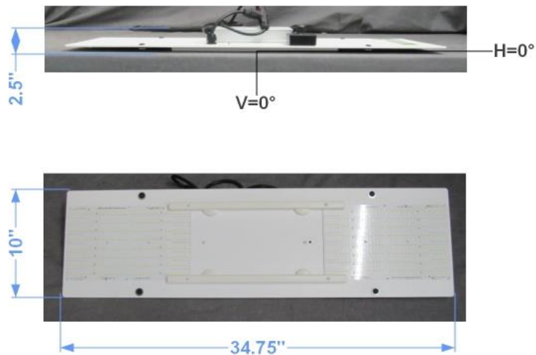
FIG. 1 LUMINAIRE
